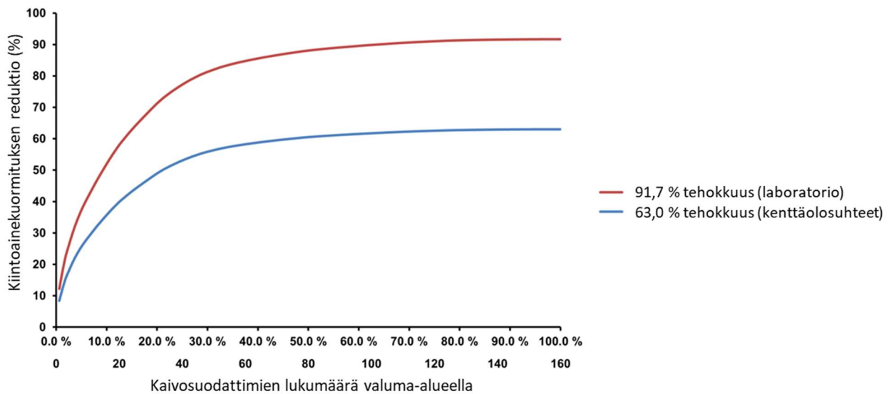
Kuva 16. Valuma-alueelta purkautuvan kiintoainekuorman reduktio kaivosuodattimien suhteellisen osuuden ja lukumäärän suhteen. Yksittäisen kaivon 91.7% suodatustehokkuus on Watecon yhteistutkimuksissa saama tulos karkealle kiintoainekselle.
